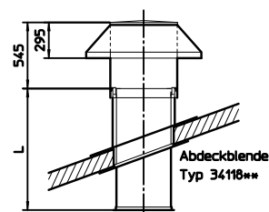
Dachsockel für Schrägdach Typ 34120**
