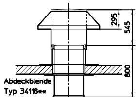
Dachsockel für Flachdach 0-4° Typ 34119
